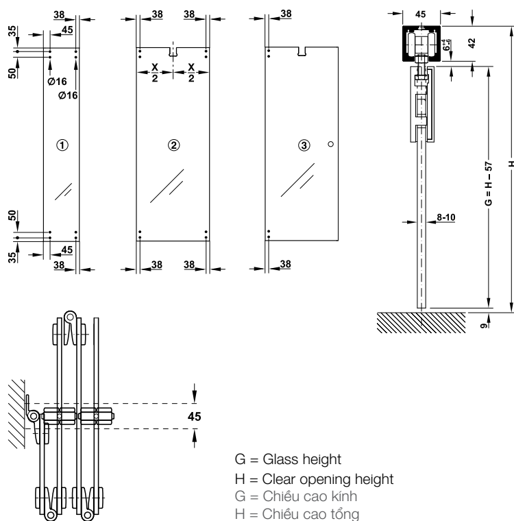
Position and type of fittings Vi trí và các loại phụ kiện
