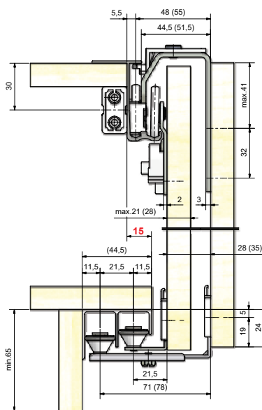
Installation dimensions Kích thước lắp đặt
