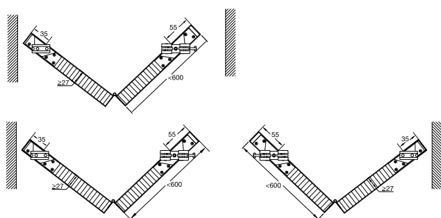
Top view installation Mặt chiếu bằng
