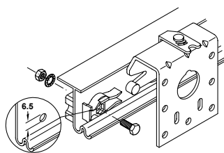
Installation/ Lắp đặt Track stopper/ Thanh chặn
