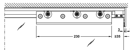
Section trolley hanger 120 kg Vị trí bánh xe treo 120 kg
