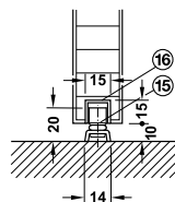
Floor guide with U-shaped guide track in door leaf and floor guide roller Dẫn hướng sàn kèm theo thanh dẫn hướng gắn cửa dạng chữ U
