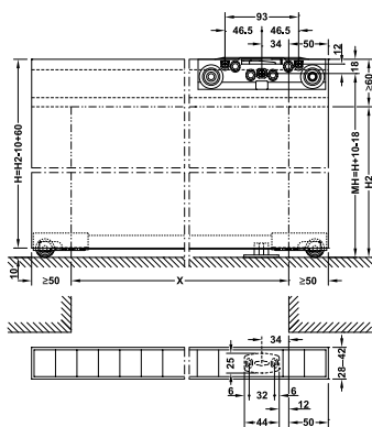
Panel preparation detail Chi tiết khoan cửa
