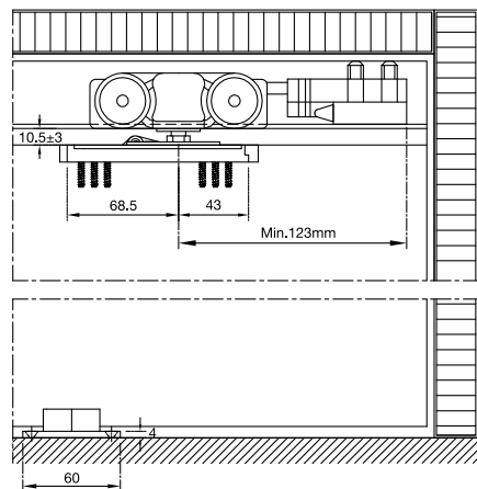
Selection guide and trolley hanger Lựa chọn dẫn hướng và bánh xe trượt
