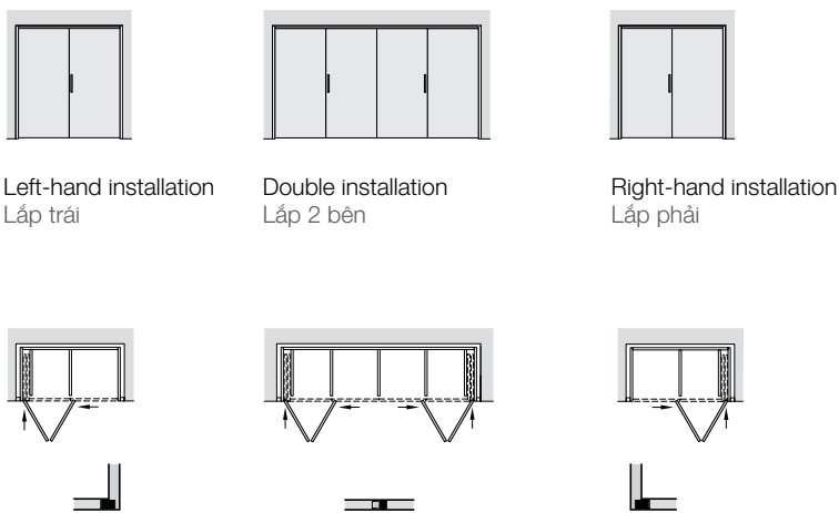
Flush door centering with magnetic centering components Giữ cửa trung tâm với nam châm
