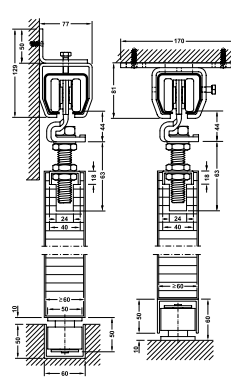
Section guide and trolley hanger 750-Q Lựa chọn dẫn hướng và bánh xe trượt 750-Q
