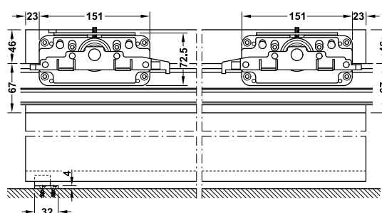
Section trolley hanger and guide Vị trí bánh xe và dẫn hướng
