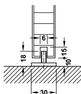
Floor guide without guide track in door leaf Dẫn hướng không gồm thanh dẫn hướng gắn cửa
