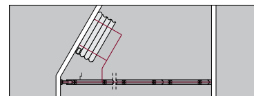
Two point suspension, cross guidance, CG (4 x) Hai điểm treo, dẫn hướng chéo, CG (4 x)
