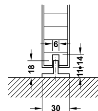
Floor guide Bas dẫn hướng
