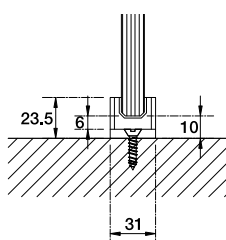
Floor guide Dẫn hướng
