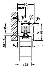
Wall installation with clip panel Treo tường với nắp che
