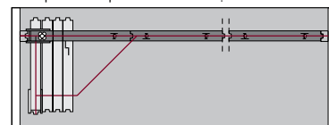
Two point suspension, forced guidance, FG Hai điểm treo, dẫn hướng bắt buộc, FG
