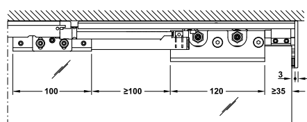
Section trolley hanger 50 kg with soft closing mechanism Vị trí bánh xe treo 50 kg với giảm chấn
