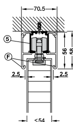
Clipping installation with clip panel Gắn trần với nắp che
