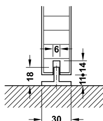
Floor guide Bas dẫn hướng
