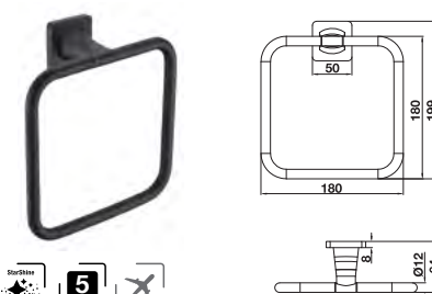
Towel ring 180x199x64mm Vòng treo khăn 180x199x64mm
