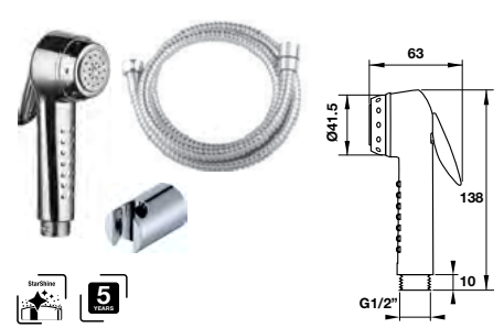
Bộ vòi xịt WC WC rinsing spray
