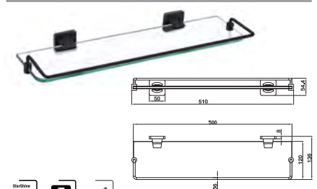
Glass shelf 510x54.4x136mm Kệ kính 510x54,4x136mm
