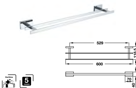
InnoSquare double towel bar Thanh treo khăn đôi InnoSquare
