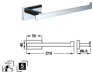
InnoSquare paper holder (excl. lid) Giá treo giấy vệ sinh không nắp che
