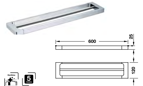
InnoGeo-S double towel bar Thanh treo khăn đôi InnoGeo-S
