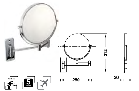
Shaving mirror Gương cạo râu
