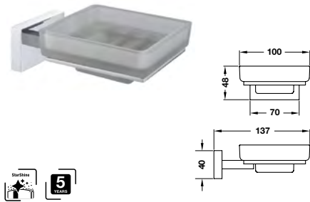
InnoSquare soap dish Đĩa đựng xà phòng InnoSquare
