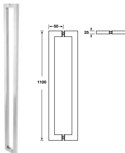
Square Pull Handle C-C 450mm Tay nắm kéo dạng vuông C-C 450mm
