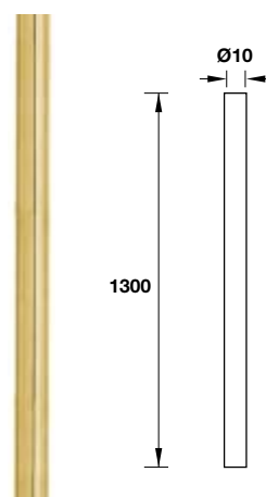
Rod for Cremone bolts brass polished PVD Thanh chốt cho bộ Cremone màu đồng bóng PVD
